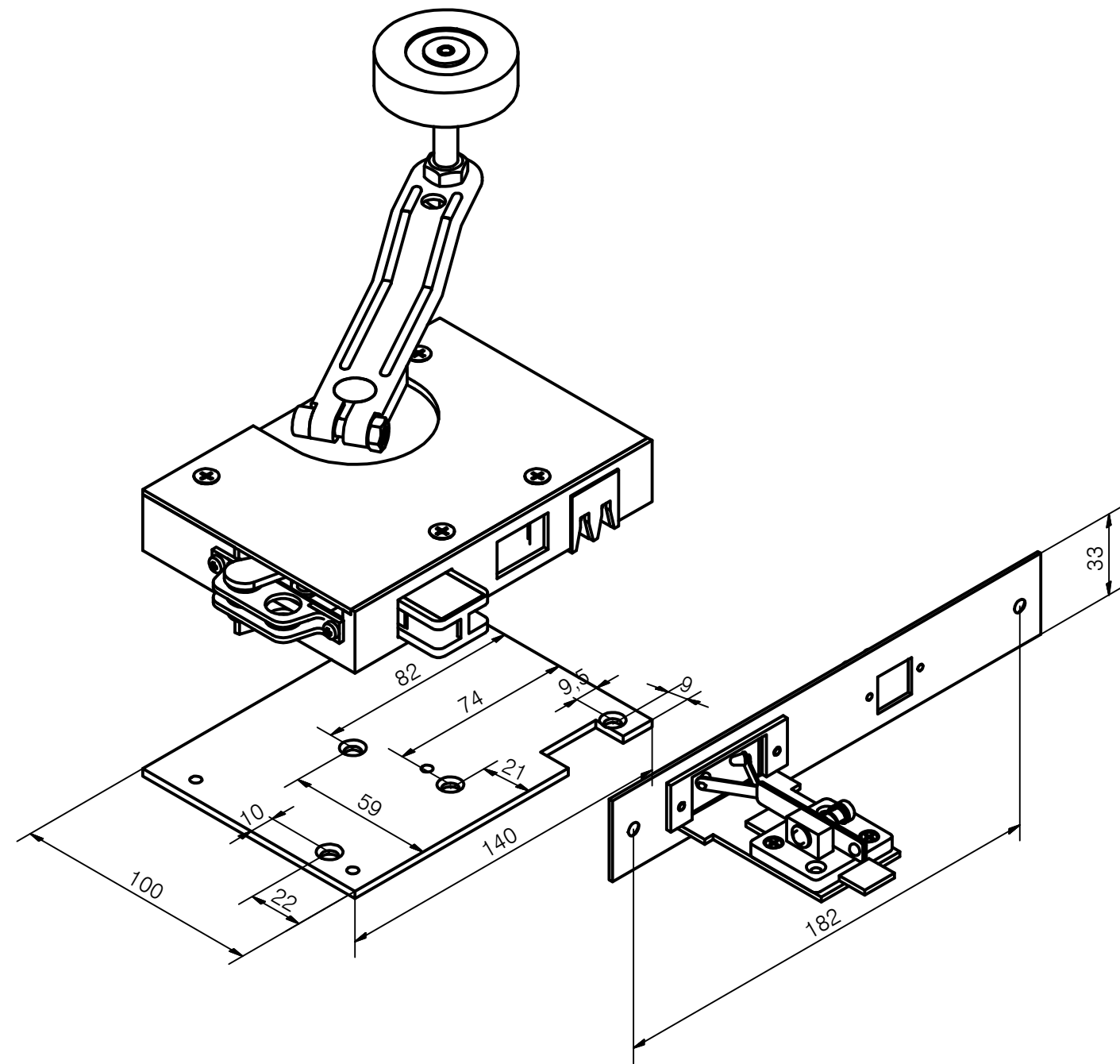
art.06.09/009600 KIT DALLAGIOVANNA SEMIAUTOMATICO EN 81
